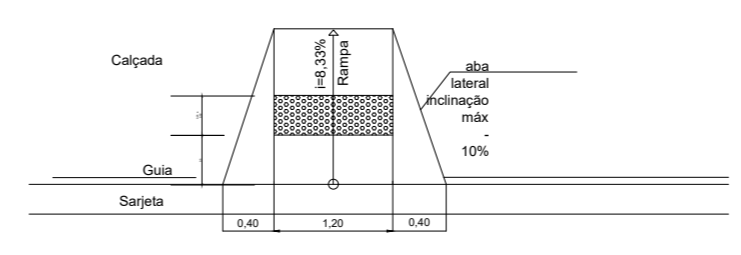
2- Detalhe rebaixamento de rampa
