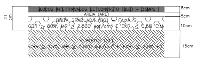
1- Detalhe execução piso intertravado
